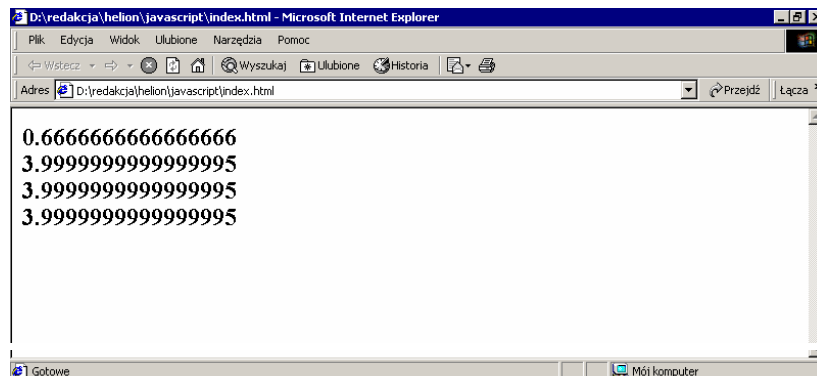
Rysunek 4.5. Efekt wykonania skryptu z ćwiczenia 4.13 w przeglądarce Internet Explorer
