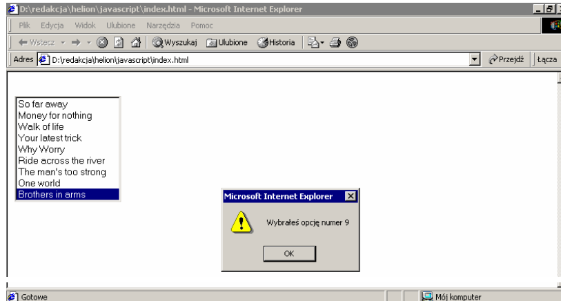
Rysunek 5.5. Obsługa listy wyboru w JavaScript
