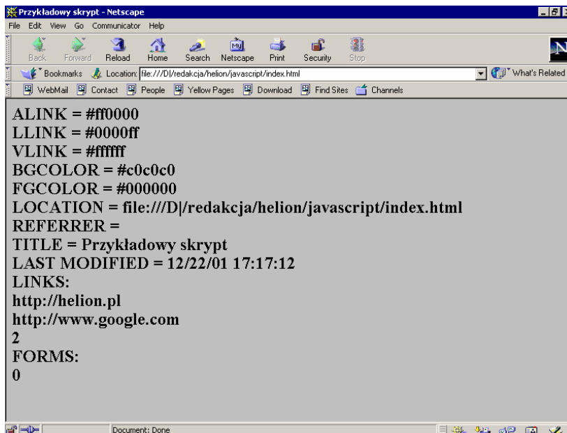
Rysunek 4.9. Efekt działania skryptu z ćwiczenia 4.16 w przeglądarce Netscape Navigator
